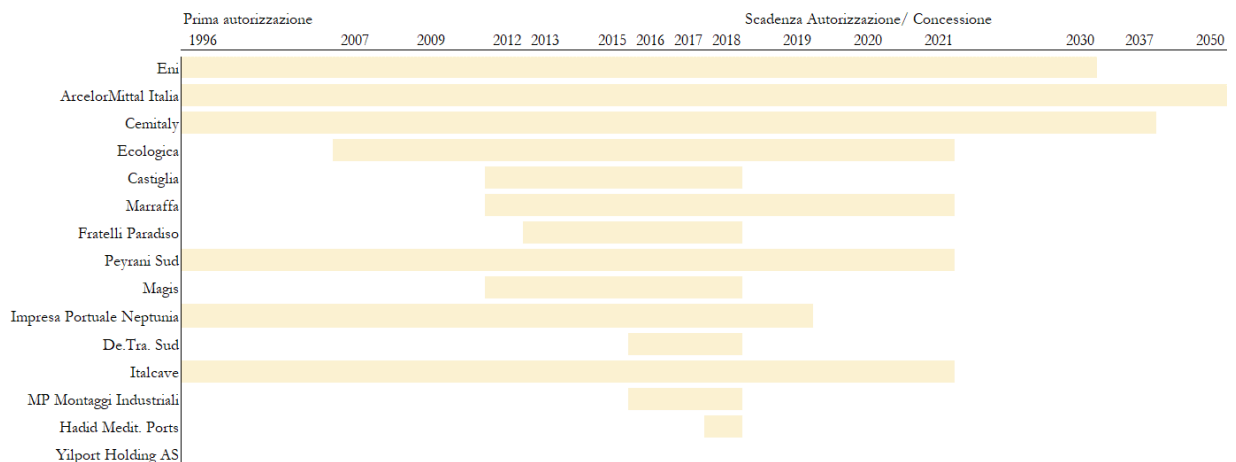
Figura 2: Data di prima autorizzazione/concessione e scadenza autorizzazione/concessione
