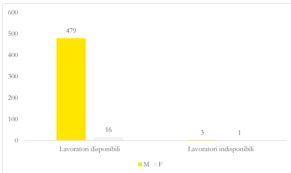
Figura 19: Lavoratori per disponibilità e sesso
