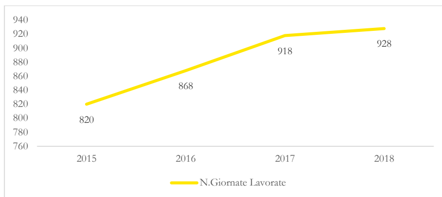
Figura 18: Trend giornate personale Compagnia
