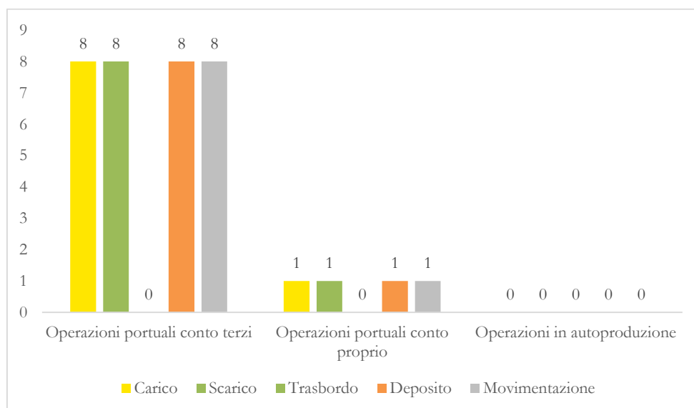
Figura 3: Autorizzazioni per Operazioni portuali nel Porto di Taranto per Modalità di erogazione
