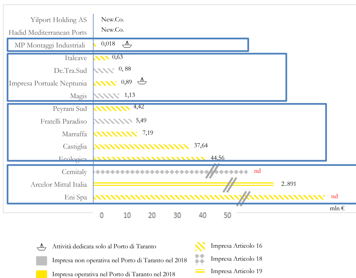
Figura 5: Imprese per fatturato (mln €), per articolo 16 - 18 - 19 L.84/94 e operatività
