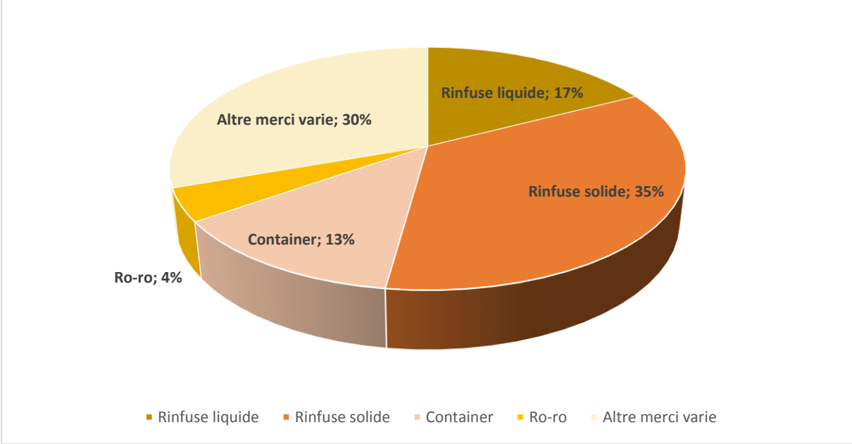
Figura 7: Diffusione segmenti di traffico tra le Imprse operanti in porto
