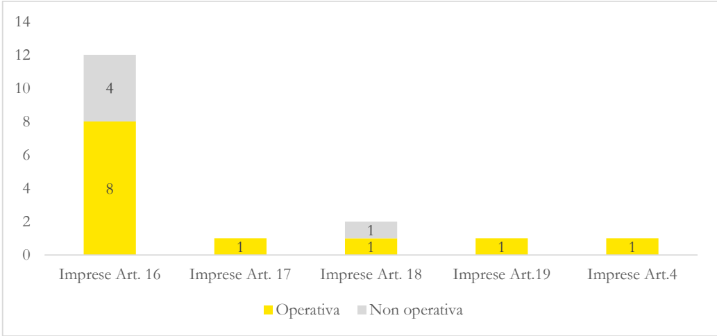
Figura 6: Imprese articolo 16,17,18,19 L.04/94, articolo 4 D.L. 243/16 che operano in Porto
