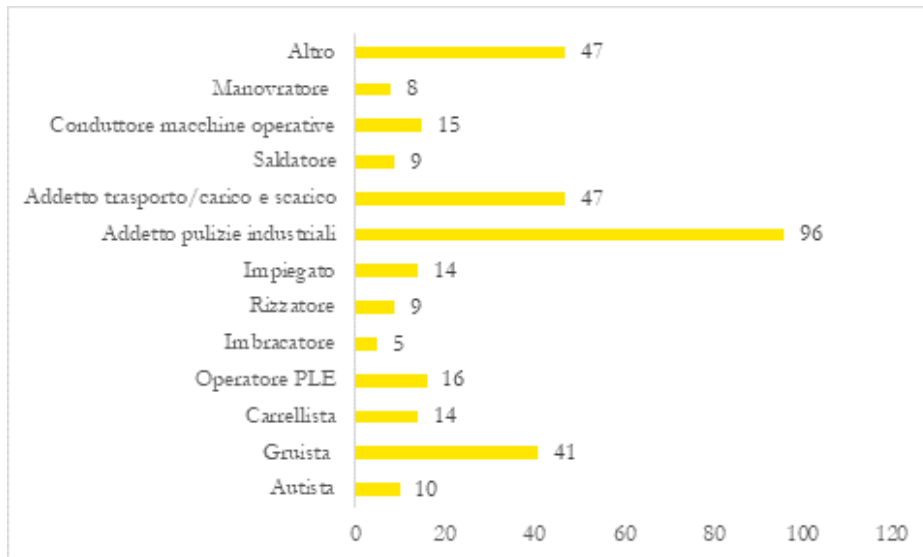
Figura 14: Mansioni più frequenti 11
