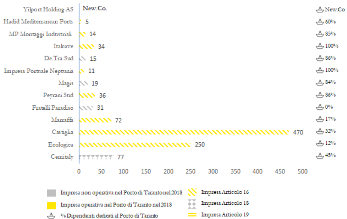
Figura 12: Lavoratori 2018 per impresa
