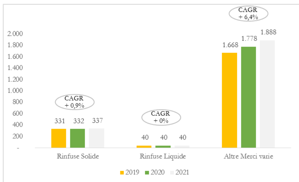
Figura 15: Volumi previsionali per segmento di traffico (valori in migliaia di tonnellate)
