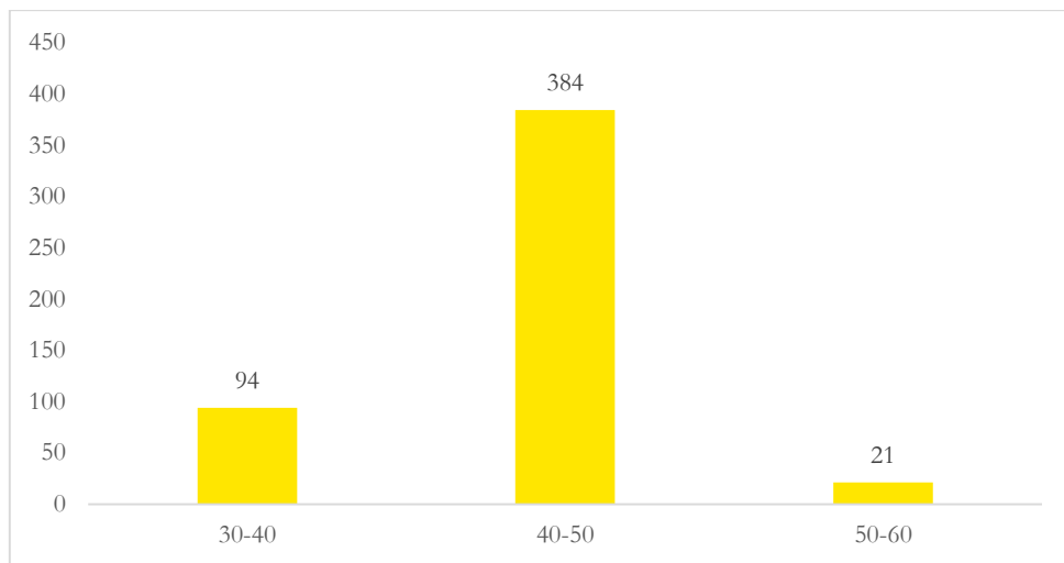
Figura 20: Lavoratori per fascia di età
