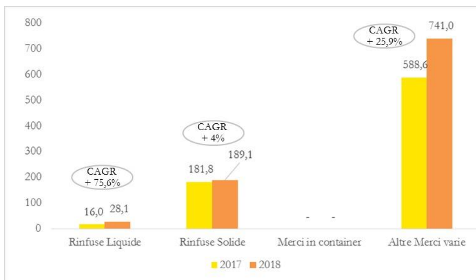
Figura 10: Volumi 2017- 2018 per segmento di traffico (tonnellate)
