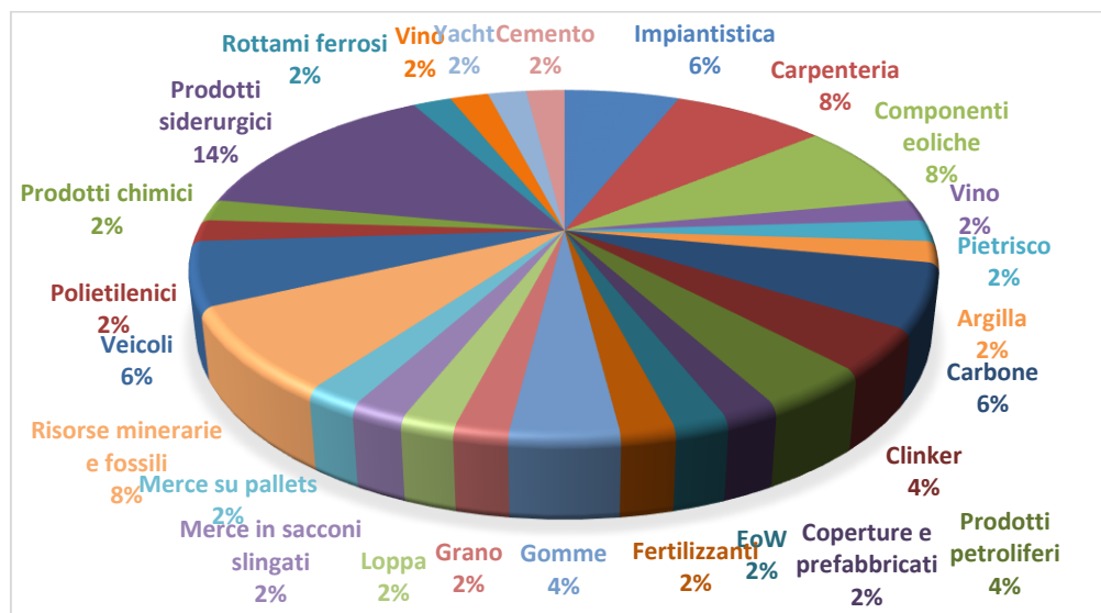
Figura 8: Categorie Merceologiche autorizzate
