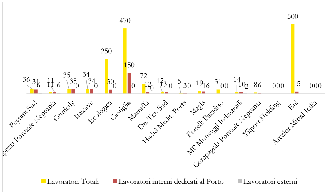
Figura 13: Mappatura lavoratori per impresa
