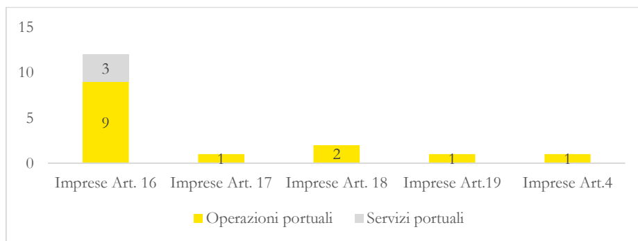
Figura 1: Imprese articolo 16,17,18,19 L.84/94, articolo 4 D.L. 243/16
