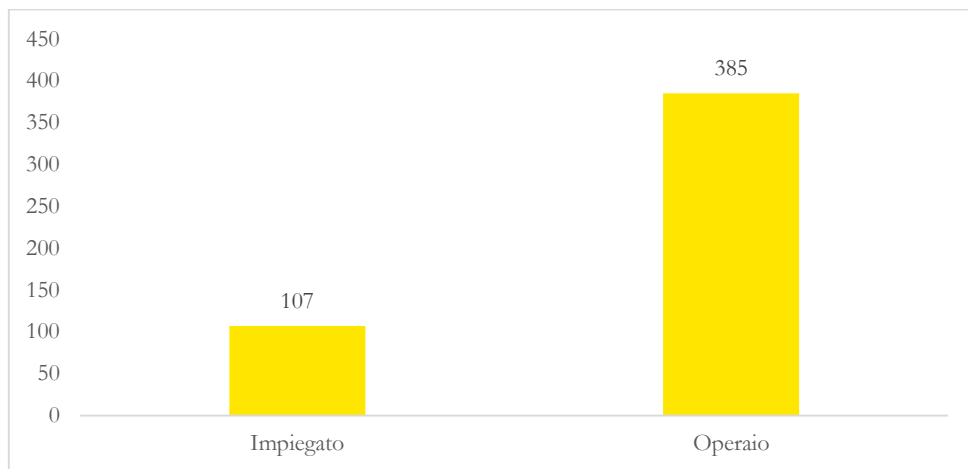
Figura 21: Lavoratori per qualifica
