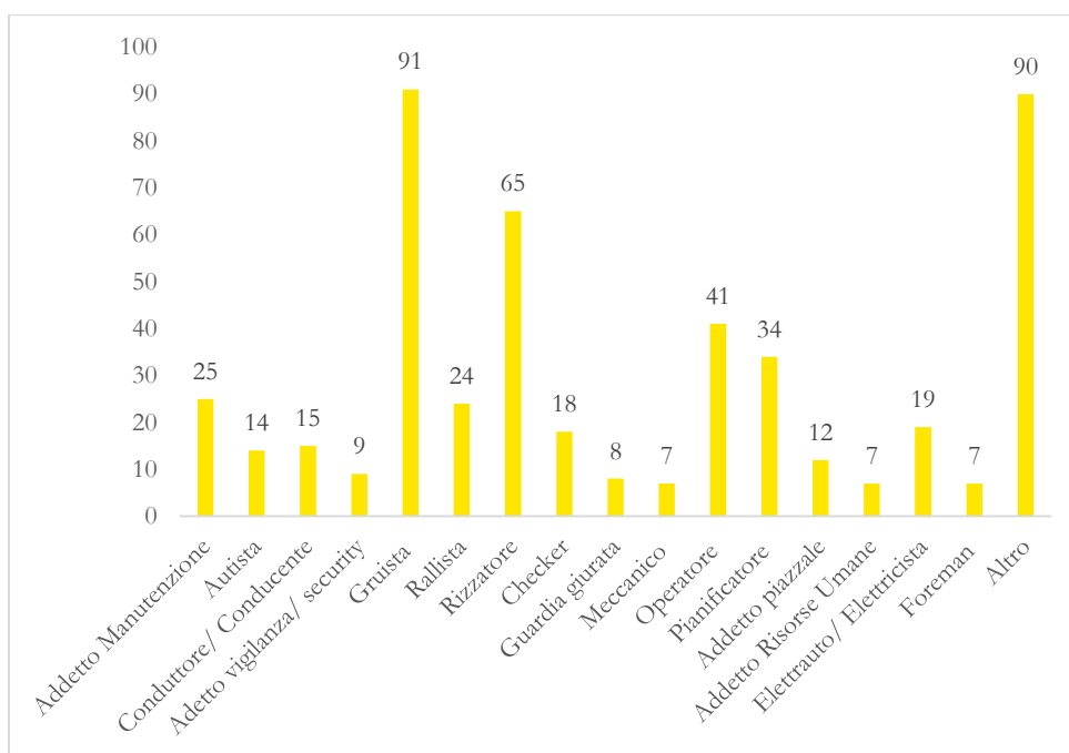
Figura 22: Lavoratori per mansione
